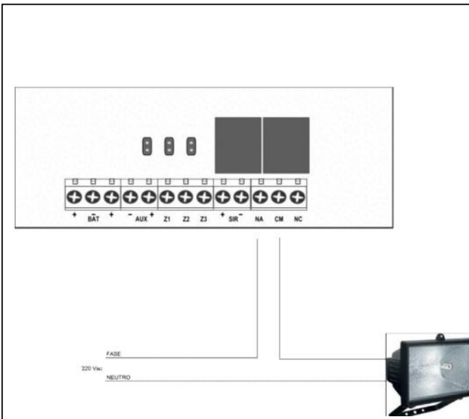
Fig. 2: Conexion directa de un reflector 300W maximo.
