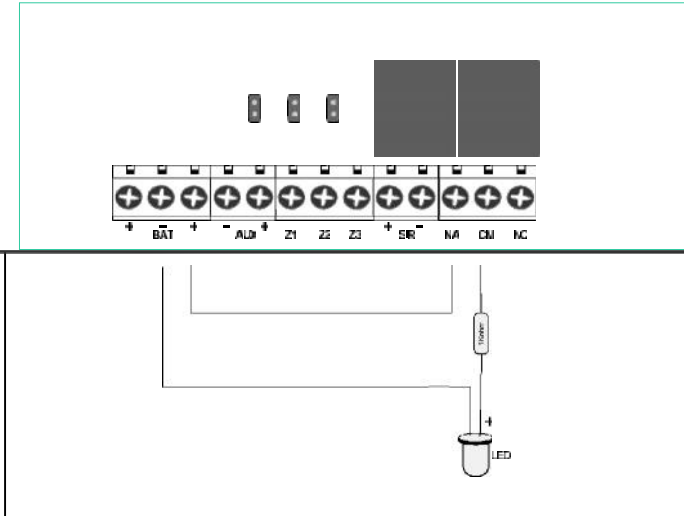
Fig. 1: Conexion de led indicador de estado.
